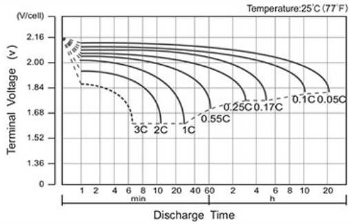
Características de la curva de descarga
