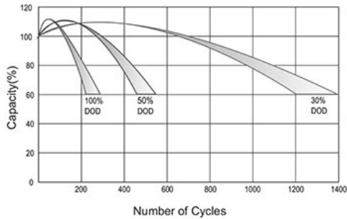
Ciclos de vida en función de la profundidad de descarga
