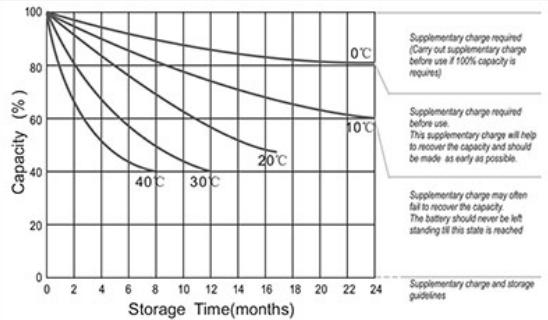
Características de almacenamiento
