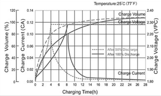
Características de la curva de carga por ciclo de uso (IU)
