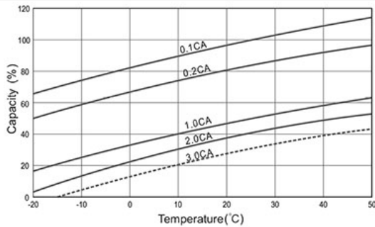
Efectos de la temperatura en la capacidad
